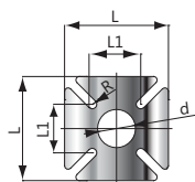
SHR-U-ES talp méretek
