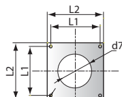
Talp méret
