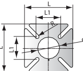
Talp méret
