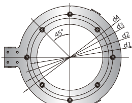
Tölcsér fedél
